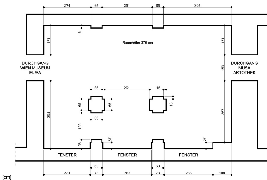
Grundriss Startgalerie
